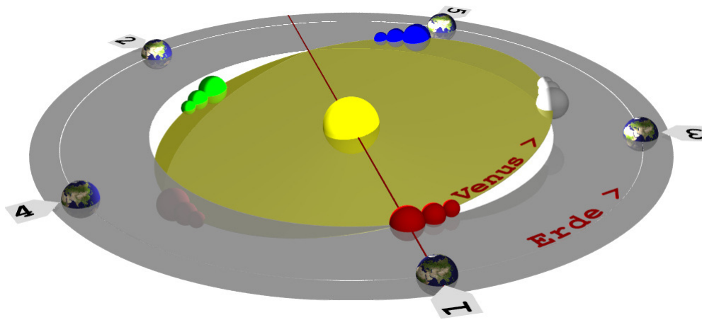
Bild 1 Schematische Bahnen von Venus und Erde. Die Orte der unteren Venus-Konjunktionen bilden ein Fünfeck. Erde und Venus erreichen die jeweils nächste Position (1-2-3-4-5) nach knapp 584 Tagen, was 1.6 Jahren oder 2.6 Venusjahren entspricht. Zu Transits kommt es nur, wenn eine Ecke in der Nähe eines der beiden Knoten zu liegen kommt. Das Schema zeigt die Situation ganz links in Bild 2 mit einem Transit an der "roten Ecke". Da sich das Fünfeck der Venus einmal in 1215 Jahren entgegen der Umlaufrichtung von Venus und Erde um die z-Achse dreht, kommt es in durchschnittlich 121.5 Jahren zu einem oder zwei Transits an der "grünen Ecke" am absteigenden Knoten, nach weiteren 121.5 Jahren zu einem oder zwei Transits an der "grauen Ecke" wieder am aufsteigenden Knoten, u.s.w.
