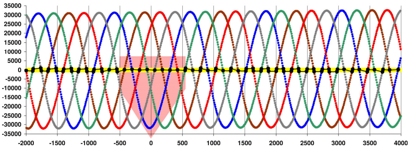
Bild 2 Untere Venus-Konjunktionen über einen Zeitraum von 6000 Jahren. x-Achse: Jahr; y-Achse: minimaler scheinbarer Abstand der Venus von der Sonnennitte ( \gamma ) in Bogensekunden. Das gelbe Band entspricht etwa der scheinbaren Grösse der Sonne, die schwarzen Punkte darauf sind die tatsächlichen Venustransits. Während der rosa Periode folgen sich Venustransits alle 121.5 Jahre, wie in Bild 1 gezeigt, abwechslungsweise am auf- und absteigenden Knoten.
